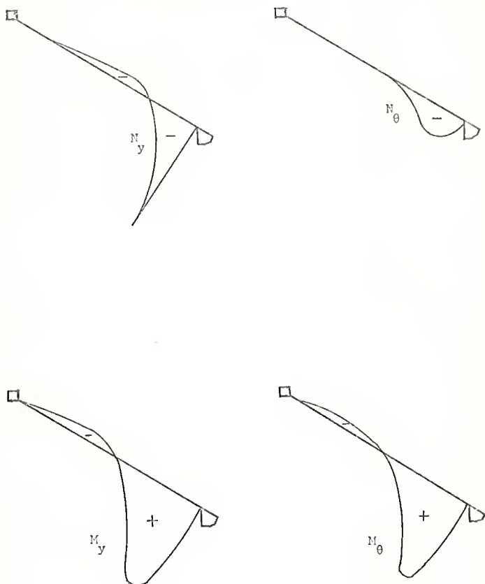
Dia. 3-3 Top edge fixed, and \Delta H = 0 , \Delta \theta = 1 at bottom edge
