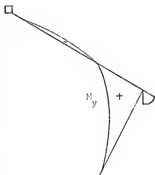
Dia. 3-5 Top edge fixed and \Delta h = 1 , \Delta \phi = 0 at bottom edge
