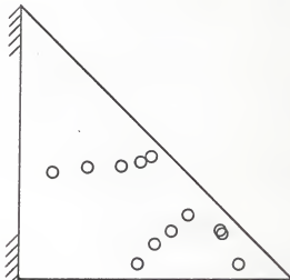
(d) Calculated nodes for mode 5
