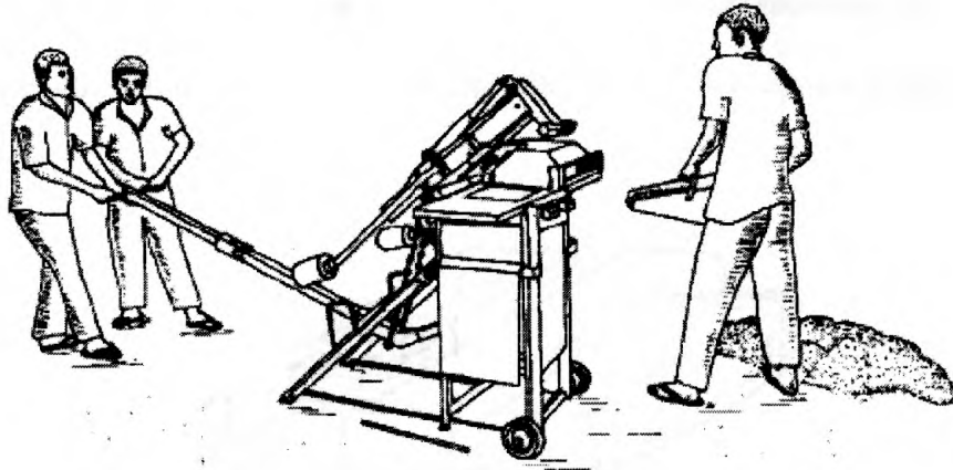
FIG. 21 CINVA-RAM
